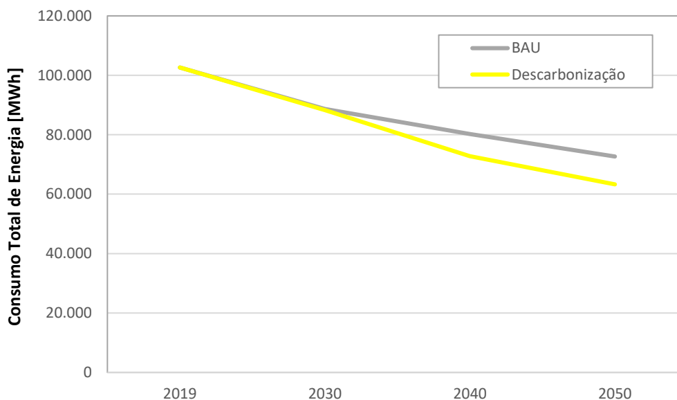
Gráfico 50: Evolução do consumo de energia (MWh), no território do concelho do Sabugal (2019-2050)
