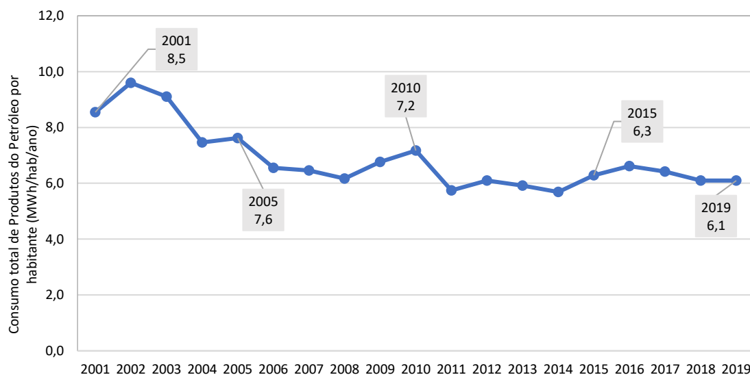
Gráfico 49: Consumo total de produtos do petróleo por habitante [MWh/hab/ano], no território do concelho do Sabugal, no período 2001-2019
