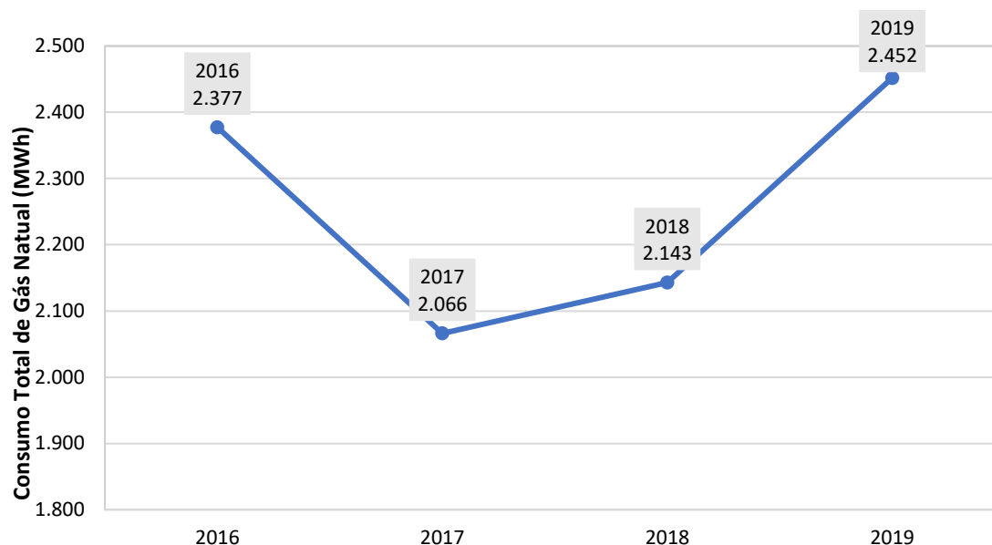
Gráfico 46: Consumo total de gás natural [MWh/ano], no território do concelho do Sabugal, no período 2014-2019
