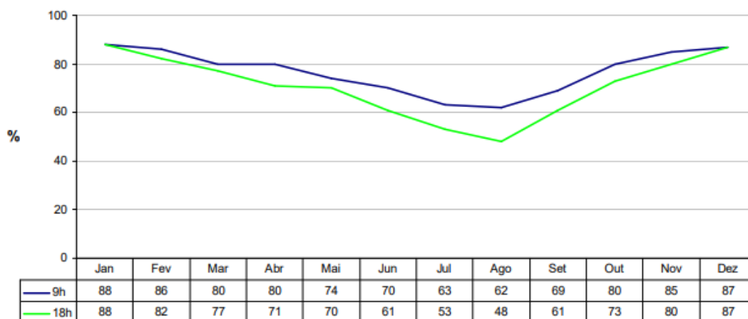
Gráfico 21: Valores médios mensais da humidade relativa do ar às 9h e 18h no concelho do Sabugal (1961-1990)
