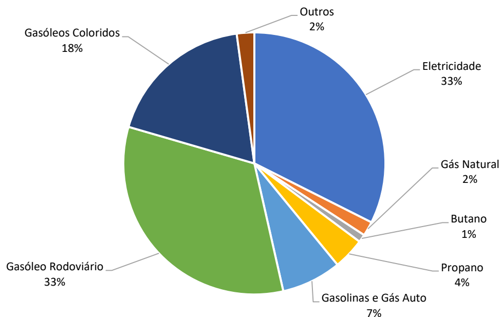
Gráfico 30: Emissões de GEE por vetor energético (%), no território do concelho do Sabugal, em 2019
