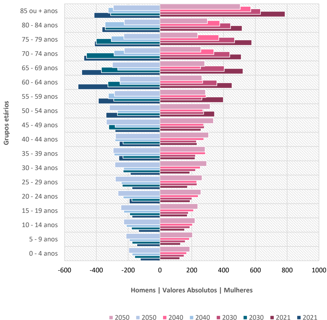
Gráfico 14: Pirâmide etária do concelho de Sabugal (2021, 2030, 2040 e 2050) – cenário baixo
