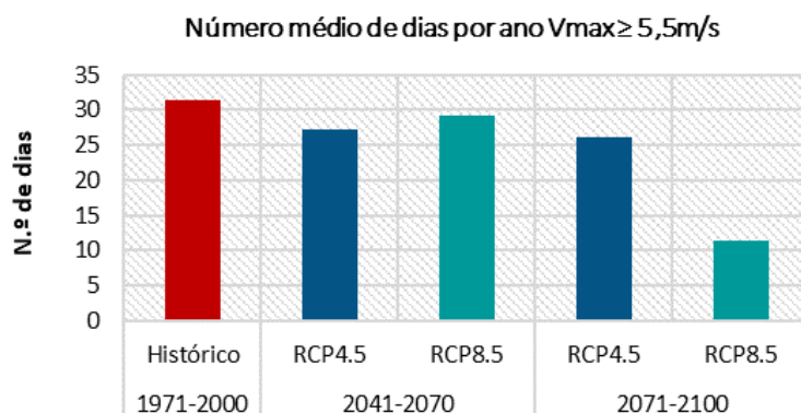
Gráfico 29: Número médio de dias com vento moderado a forte, ou com intensidade superior [modelo 2]
