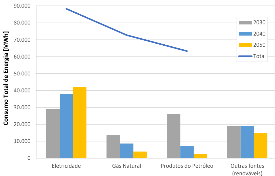
Gráfico 51: Evolução do consumo de energia (MWh), por vetor energético, no território do concelho do Sabugal, segundo o cenário de descarbonização (CD) (2030-2050)
