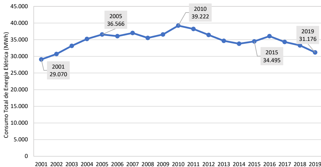
Gráfico 44: Consumo total de energia elétrica [MWh/ano], no território do concelho do Sabugal, no período 2001-2019
