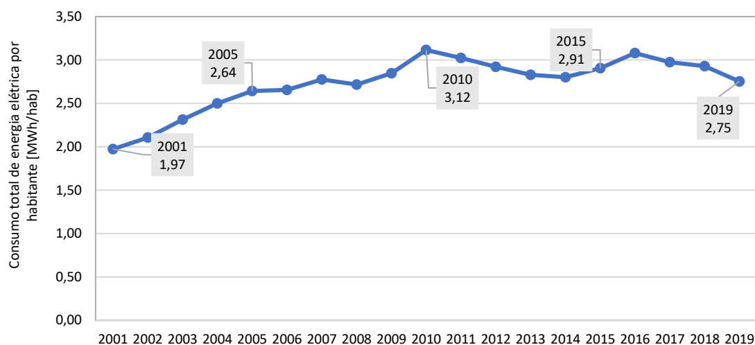
Gráfico 45: Consumo total de energia elétrica por habitante [MWh/hab/ano], no território do concelho do Sabugal, no período 2001-2019
