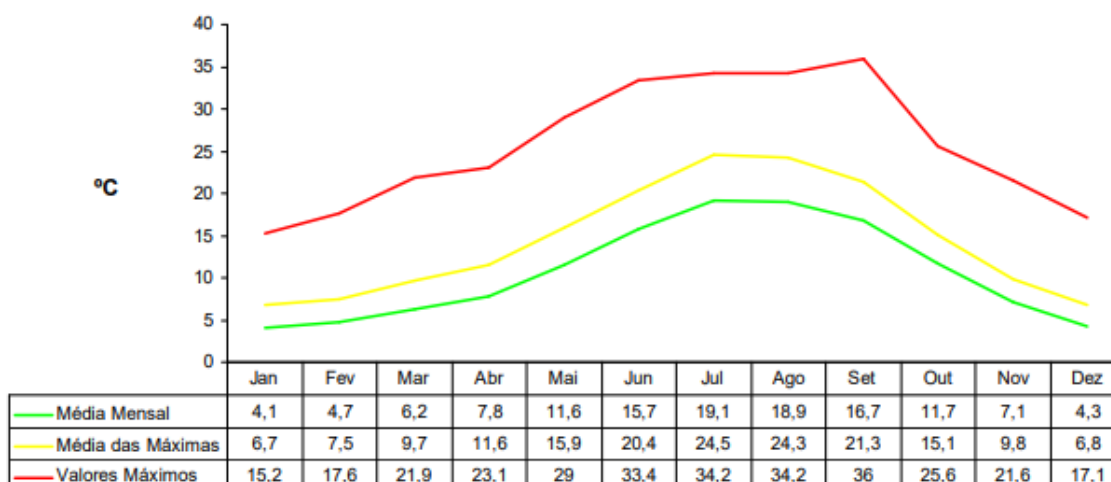
Gráfico 20: Valores mensais da temperatura média, média máxima e valores máximos no concelho do Sabugal (1961-1990)
