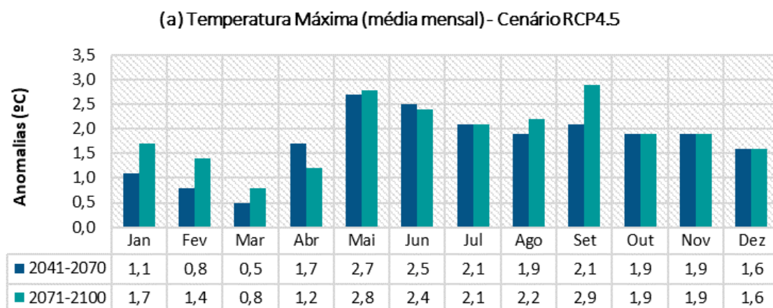
Gráfico 24: Anomalias da média mensal de temperatura máxima 4
