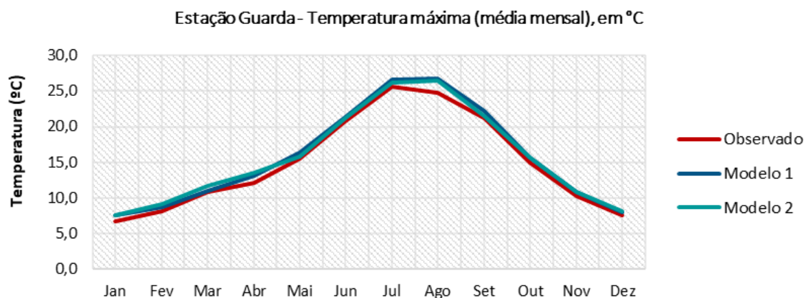
Gráfico 23: Comparação entre os valores observados (IPMA) e os modelados para o clima presente 3
